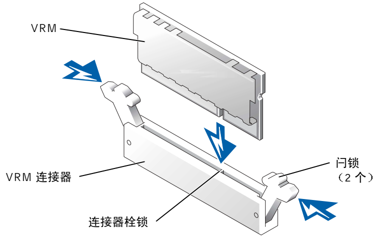
图 2-2：安装 VRM
